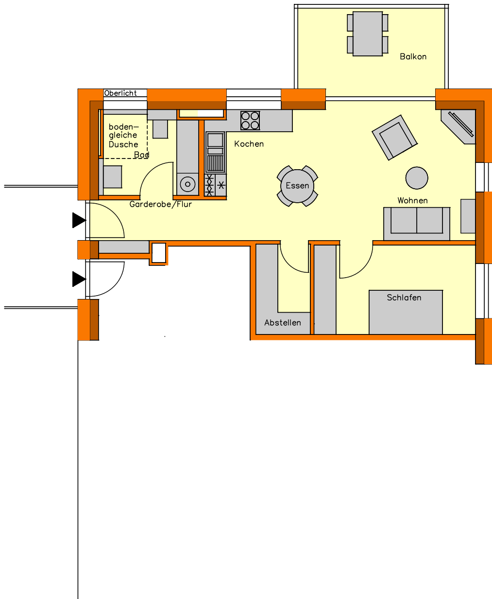
Grundriss M 1:100
