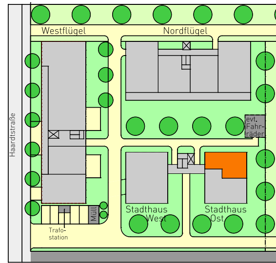
Lageplan 1. OG M 1:1000
