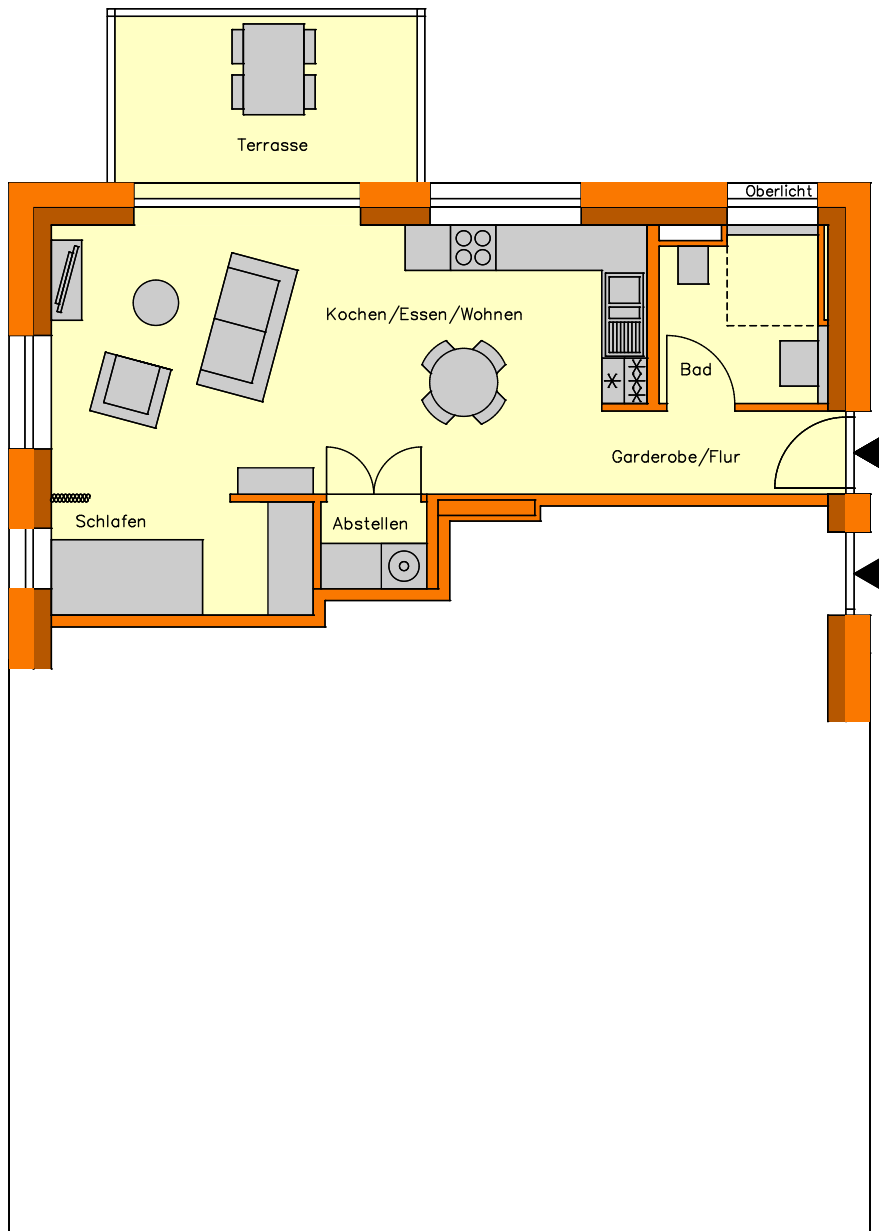
Grundriss M 1:100
