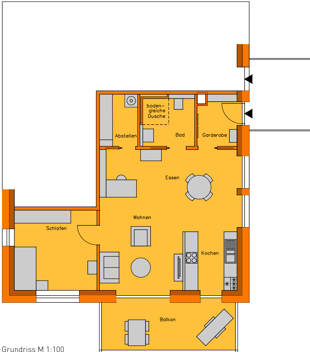
Grundriss M 1:100
