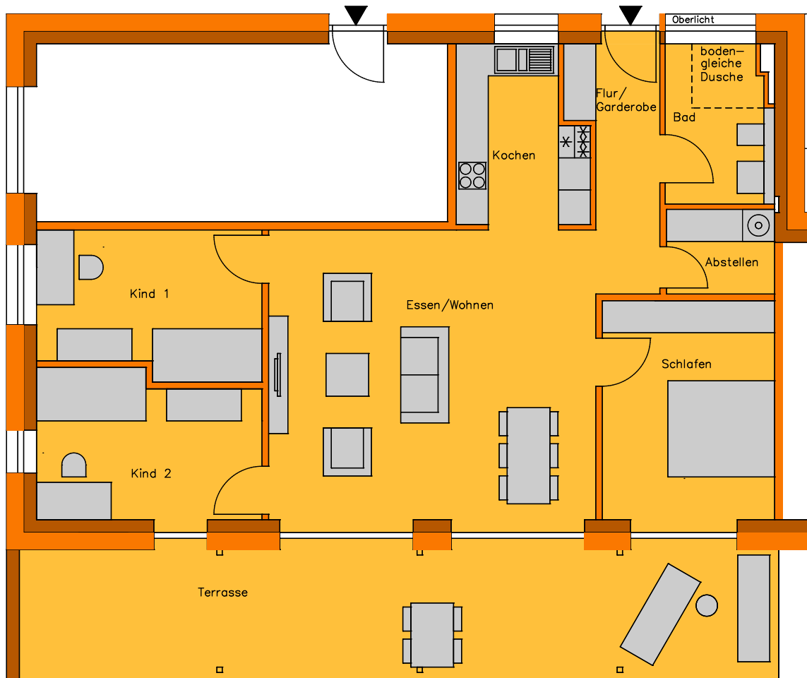
Grundriss M 1:100
